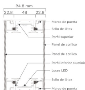
Perfil puerta aluminio
